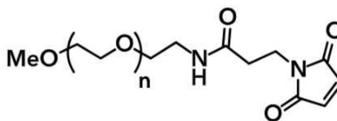
mPEG
