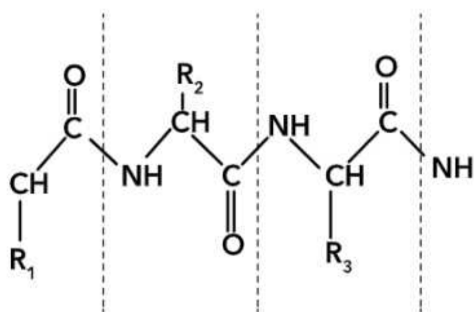
Peptide
